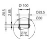
Dettaglio B
